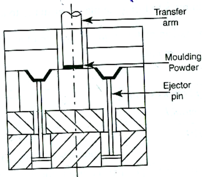
Fig. 5.10. Transfer moulding
